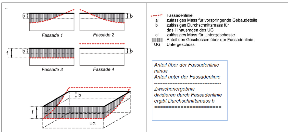
Skizze zur Figur 6.2 zum Durchschnitmass b von 80 cm gemäss Anhang 2 BauV
