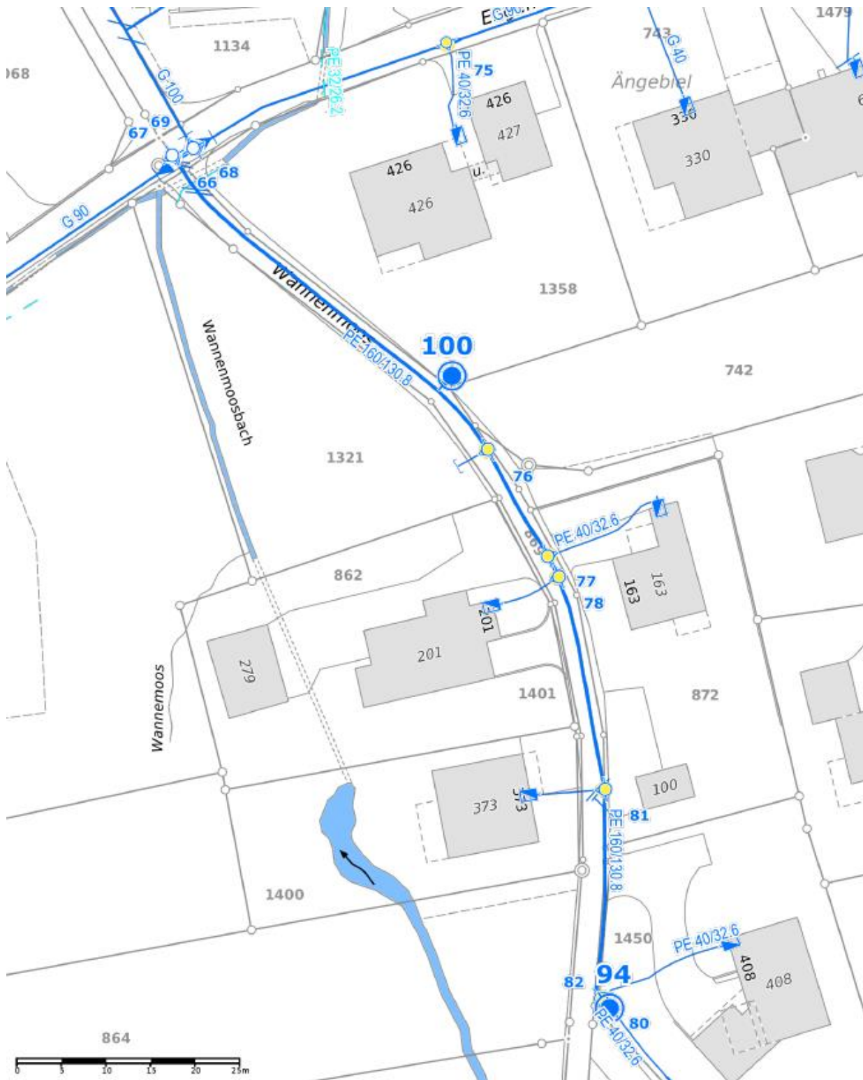
Situation Wasserleitungserweiterung "Wannemoos"
