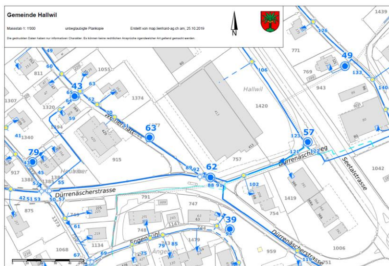
Situation Wasserleitungsverlegung Dürrenäscherstrasse/Dürrenäscherweg
